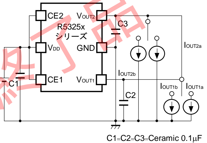
図-4 負荷過渡応答測定回路
