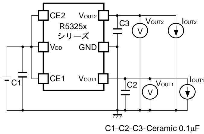
図-1 基本測定回路
