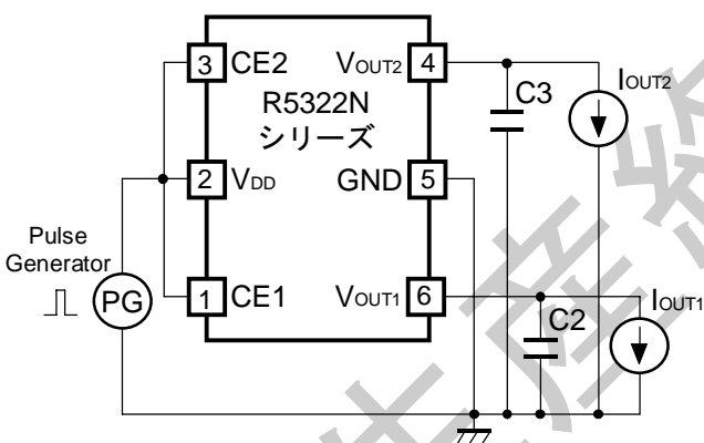
図-3 リップル除去率、入力過渡応答測定回路
