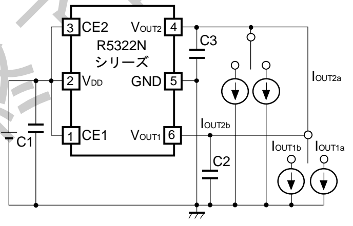
図-2 消費電流測定回路
