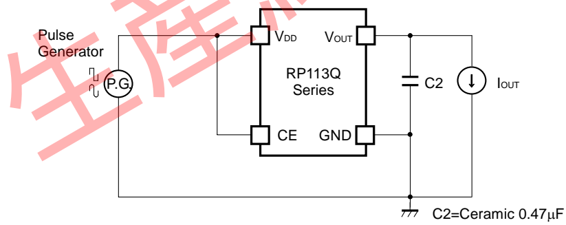
リップル除去率測定回路
