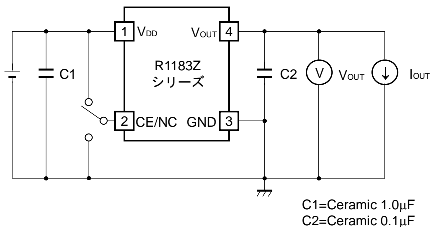
基本測定回路
