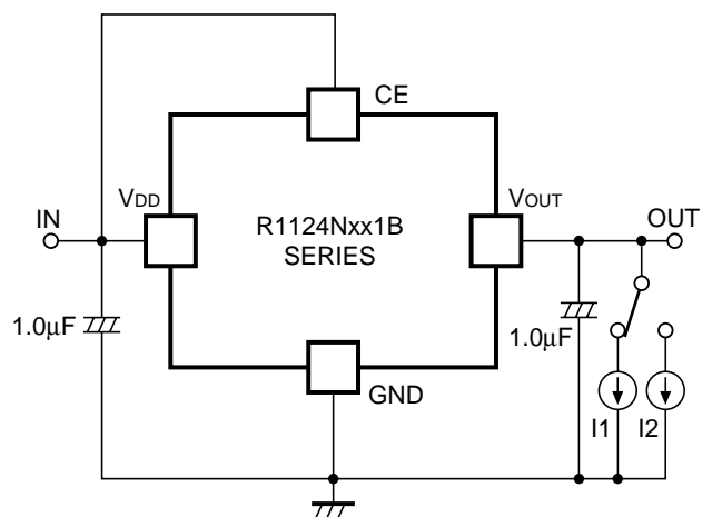
図-4 負荷過渡応答測定回路
