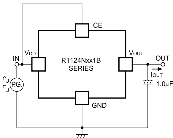
図-3 リップル除去率、入力過渡応答特性測定回路
