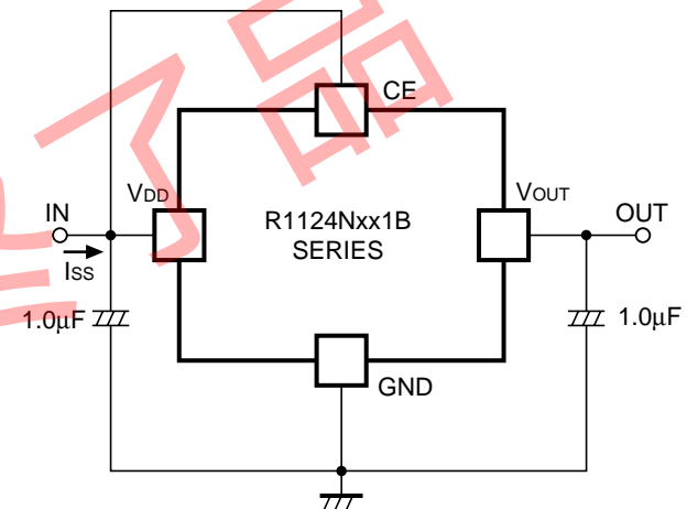
図-2 消費電流測定回路
