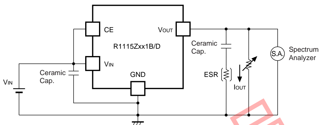
R115Zxx1B/D ノイズ測定回路
