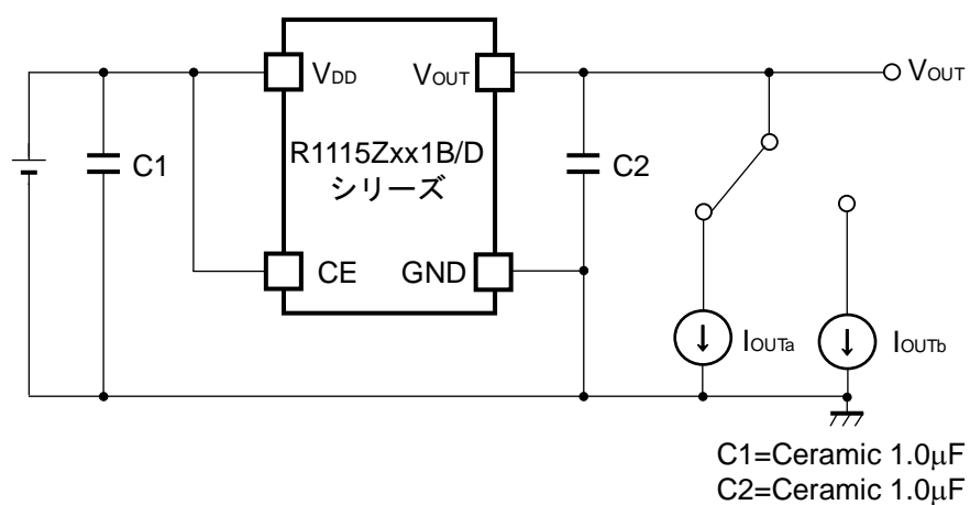
負荷過渡応答測定回路
