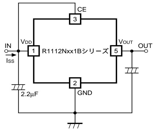
図-2 消費電流測定回路
