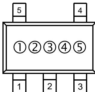
SOT-23-5 マーキング図
