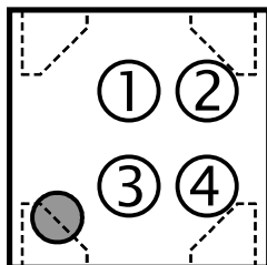
DFN(PLP)1010-4B マーキング図
