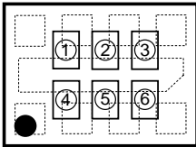
RP153LxxxA シリーズ
