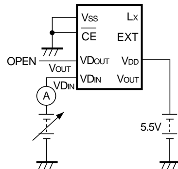
測定回路 5
