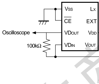
測定回路 2
