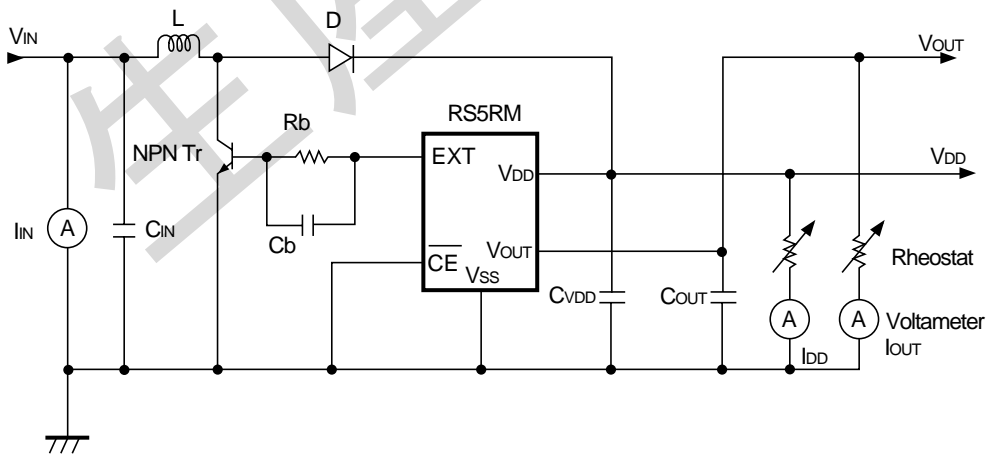
測定回路 7
