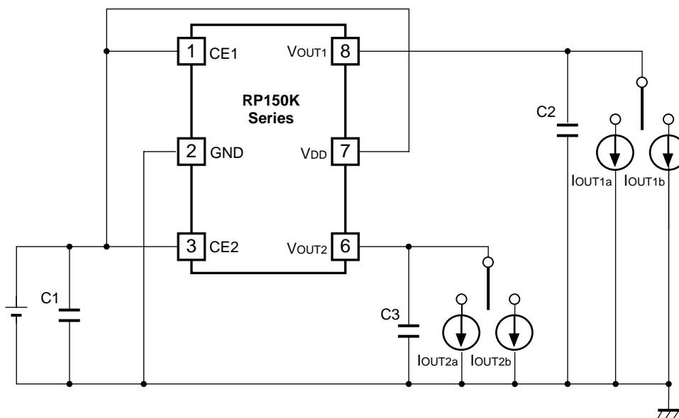
負荷過渡応答測定回路
