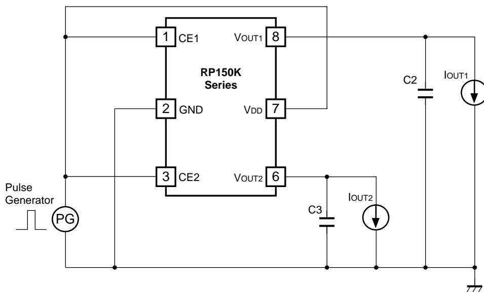
リップル除去率測定回路
