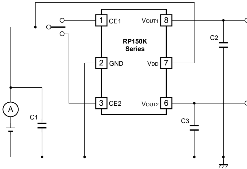
消費電流測定回路
