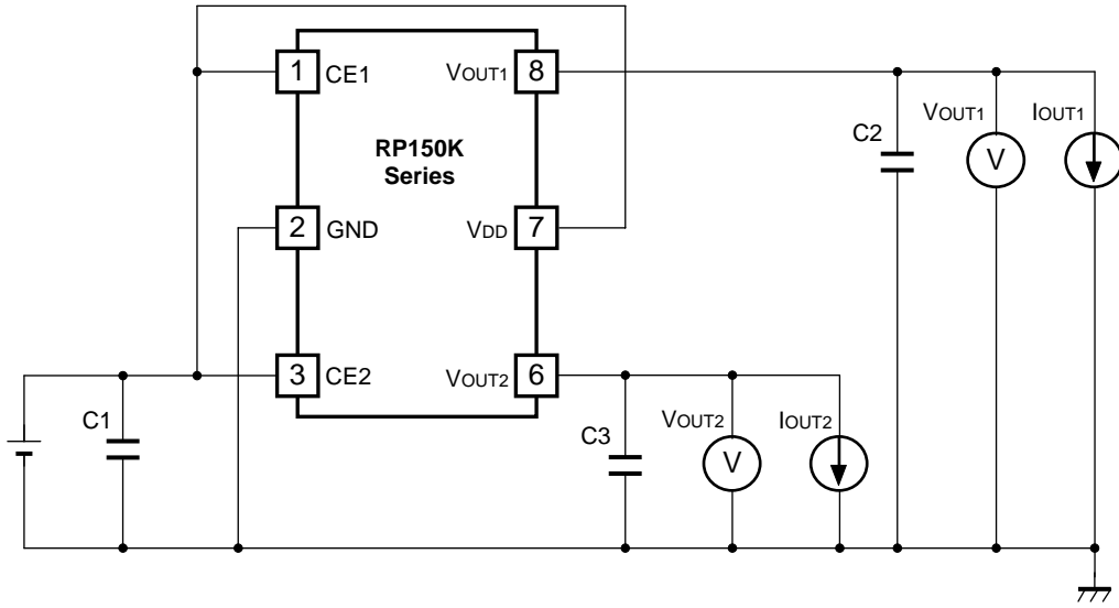
基本測定回路
