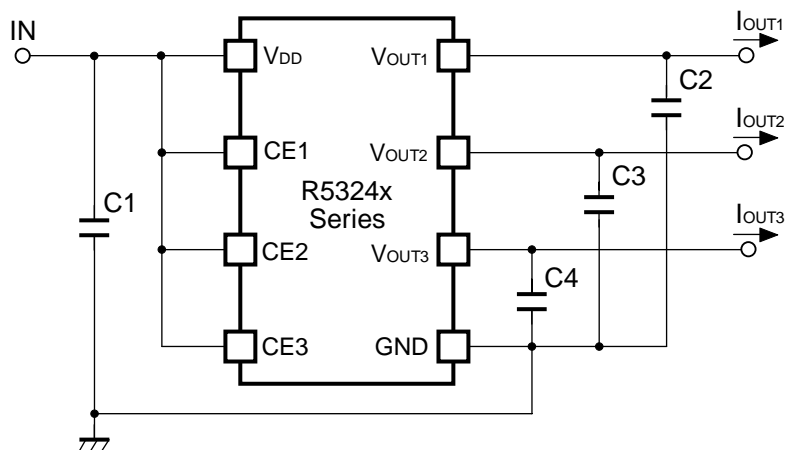
基本測定回路
