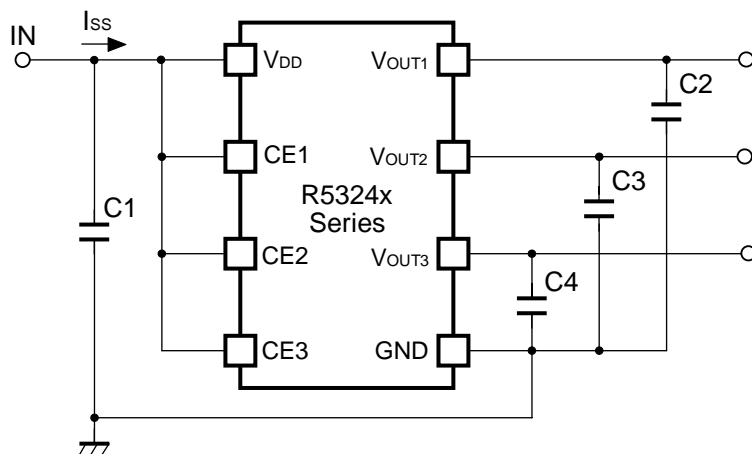
消費電流測定回路
