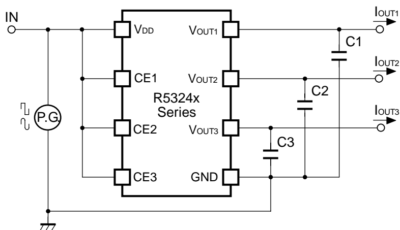
リップル除去率、入力過渡応答特性測定回路
