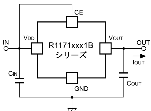
基本測定回路
