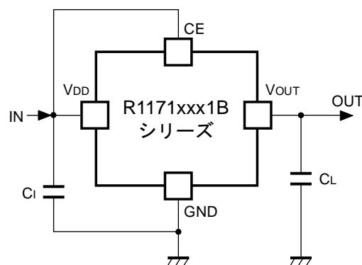
R1171Sxx1B 基本回路例
