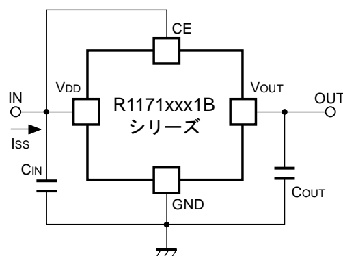
消費電流測定回路
