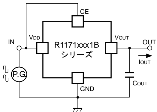
リップル除去率、入力過渡応答特性測定回路
