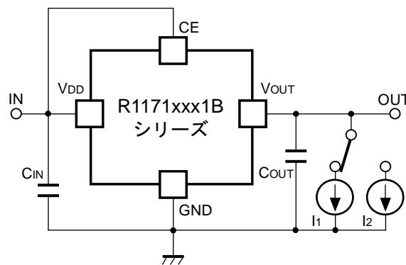
負荷過渡応答測定回路
