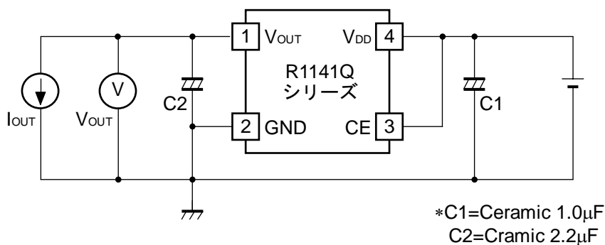
基本測定回路
