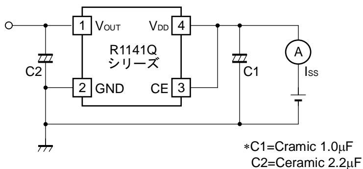
消費電流測定回路
