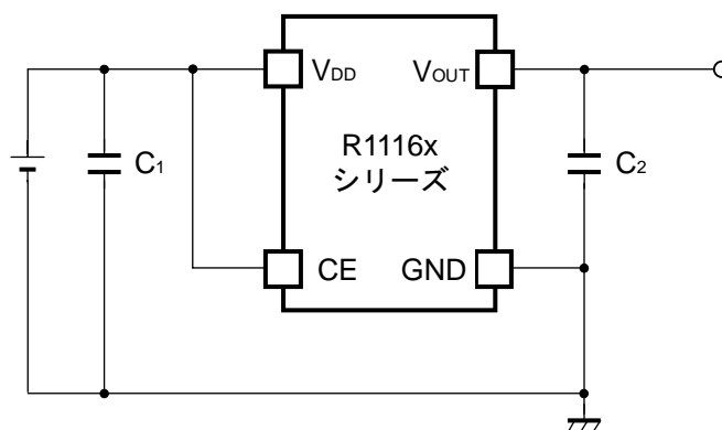
基本回路例
