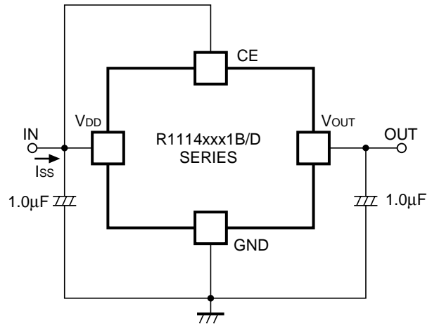
図-2 消費電流測定回路
