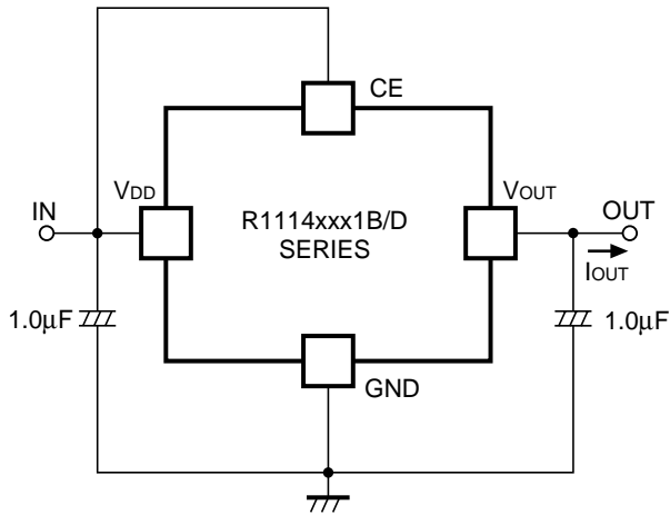
図-1 基本測定回路
