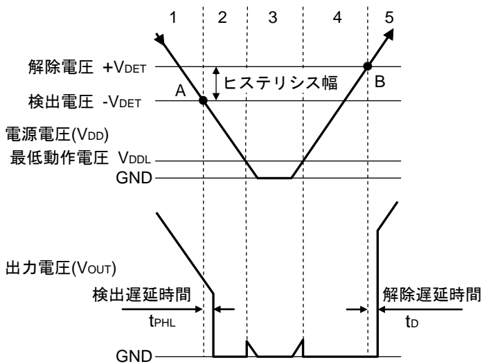
図 2. 動作状態説明図
