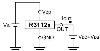
Pch ドライバ出力電流測定回路
