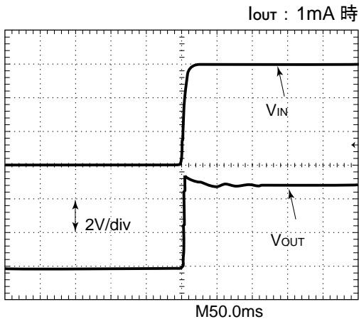
《R1210N502D》 ( V_{IN} : 0V \rightarrow 3.0V )
