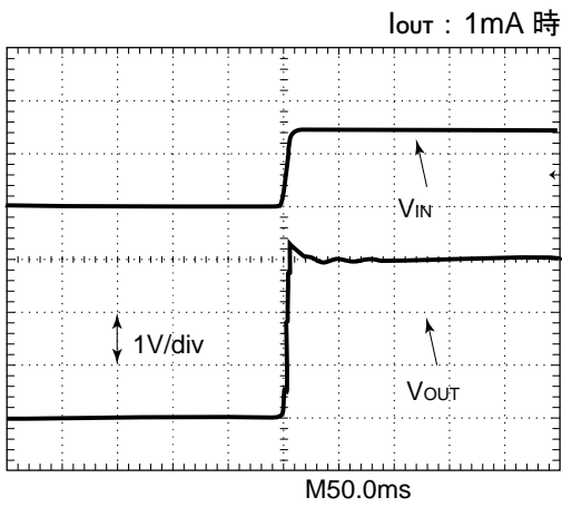
《R1210N302C》 ( V_{IN} : 0V \rightarrow 1.5V )
