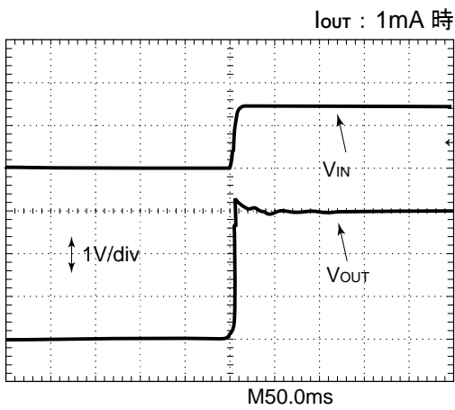
《R1210N302D》 ( V_{IN} : 0V \rightarrow 1.5V )
