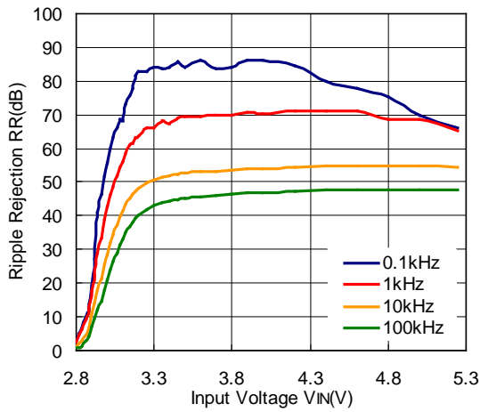
RP202x28xx (Auto ECO FAST Mode)
