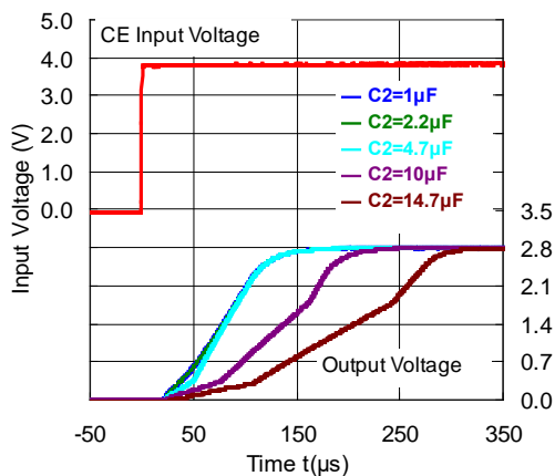
RP202x28xx VIN=3.8V, IOUT=0mA
