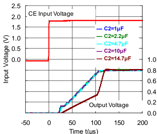
RP202x08xx VIN=1.8V, IOUT=0mA
