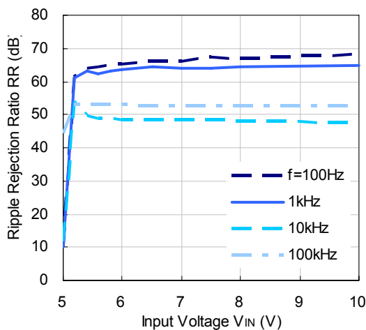
R1511x050B (I OUT =1mA)
