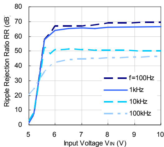
R1511x050B (I OUT =100mA)
